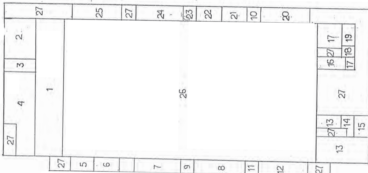
地下2階平面図 1:500
